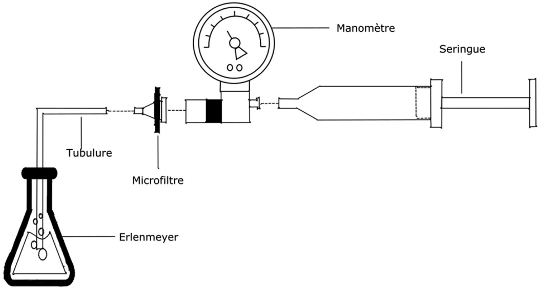
Figure 1. Montage du test du point de bulle
